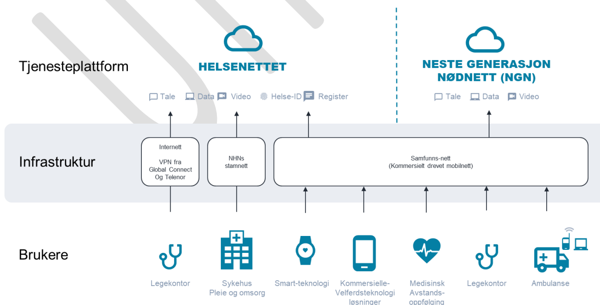
Figur 2 Illustrasjon av samhandlingsbehov ved neste generasjons nødnett
